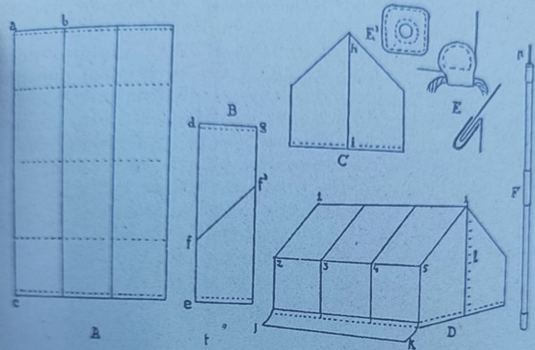
Fig. 31. — Confección de la tienda de campaña. — A: tres tiras de tela, cosidas, 1 m de ancho ( a b ) y 5 m de largo ( a c ). B: partes delantera y posterior de la tienda: se corta según la línea f f' dos tiras de tela de d e = 3 m y d g = 2 m; d f = 1,90 m, y g f' = 1,10 m, ambas piezas cortadas ya, se dejan libres (para la parte delantera) o se cosen como indica C línea h i , para la posterior. La pieza A y las dos C se cosen como indica D. En torno de la tienda, excepto por la parte delantera, y siguiendo una línea a 1 dm de distancia de su borde inferior se cose por la parte externa una banda de arpillera (unos 30 cm de ancho y 8 m de largo, j k ). En los vértices 1 y 1 de la tienda se cosen dos rodajas de cuero E' , con pequeño orificio central para dejar paso a los pivotes de los palos de la tienda. En los puntos 2, 3, 4 y 5 de la arista lateral de la tienda y en los simétricos de la opuesta se cosen abrazando la tela unas tiras dobladas de cuero (E) a las cuales se atarán las cuerdas que han de sujetar la tienda. F representa uno de los dos palos de la tienda, que han de tener 1,80 m; el pivote p basta que sobresalga unos centímetros; ha de ser un poco más largo si la tienda ha de llevar doble cubierta. Las dos mitades de la parte delantera destinada a puerta pueden cerrarse con botonadura o con cintas. (Original)
